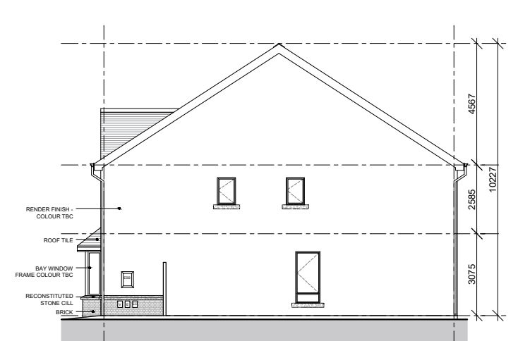
8 Side Elevation 0400
