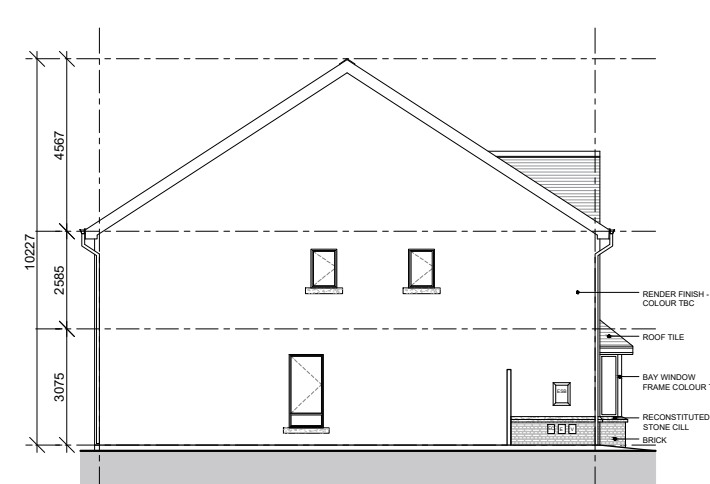
7 Side Elevation 0400
