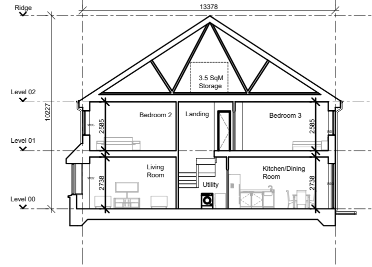
4 Section 0400
